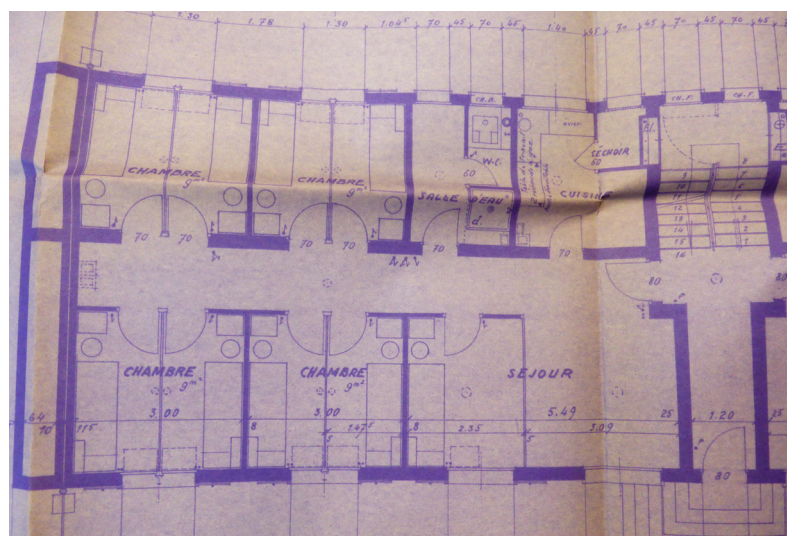
Plans des deux types de logements
