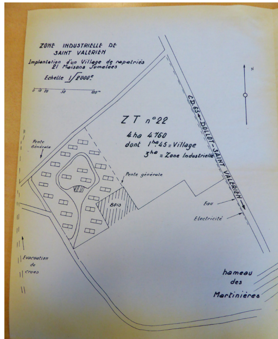
Localisation et plan du projet de l'Oasis 478
