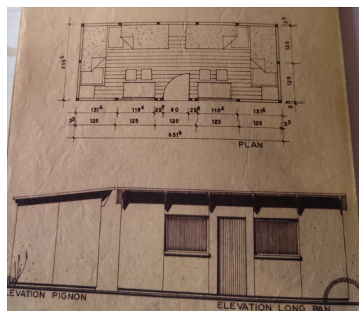
Modèle et plan d'une baraque pour 8 occupants 559
