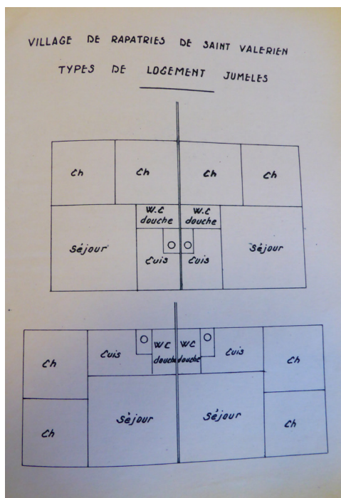
Plans des F3 jumelés 490
