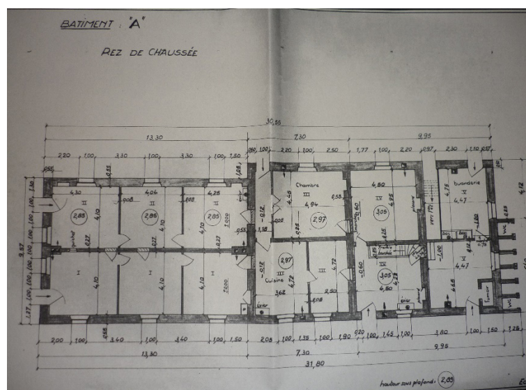
Plan de l'intérieur du bâtiment principal (AD de Moselle 297 W 30).
