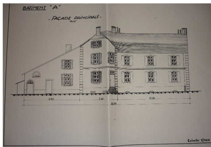
Plan de la façade principale (AD de Moselle 297 W 30).
